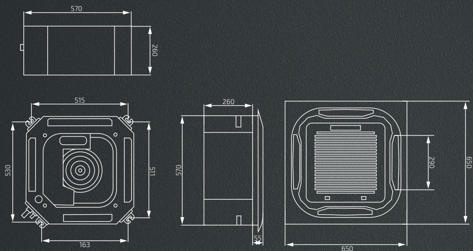
FF36/43/50CC-2PA1
